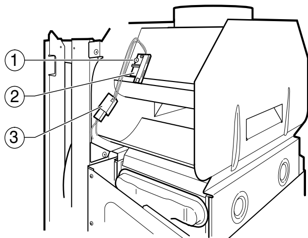
obr. 39 Snímač pro sledování spalin
