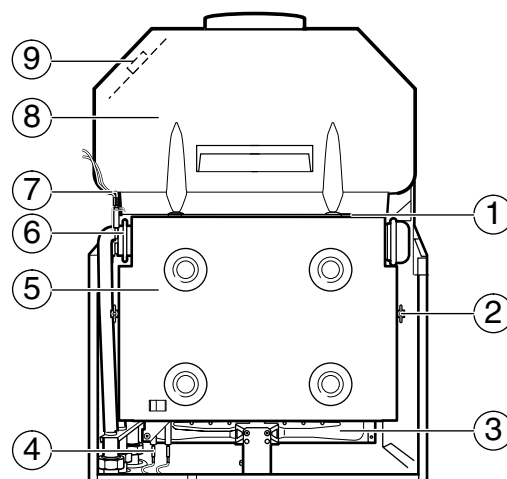
obr. 38 Komponenty vnitřního pláště
