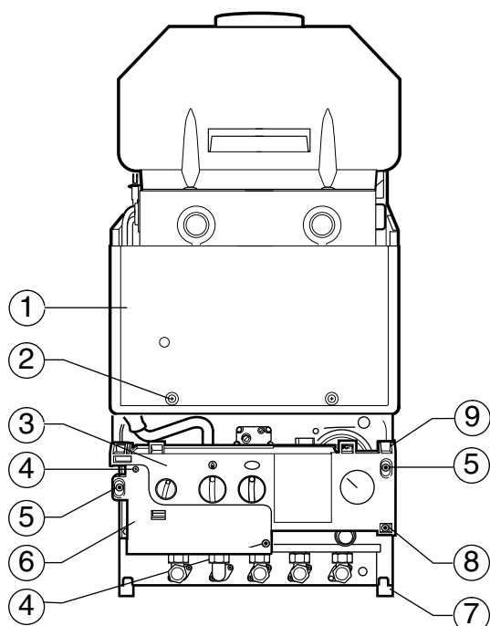
obr. 36 Vnitřní plášť a upevnění modulu
