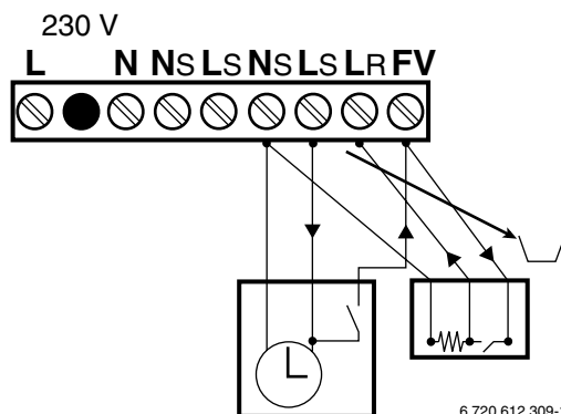
obr. 17 Připojení pokojového termostatu a programovací jednotky (odstraňte propojku mezi LS a LR)
