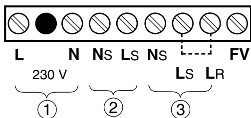
obr. 13 Připojení k elektrické síti
