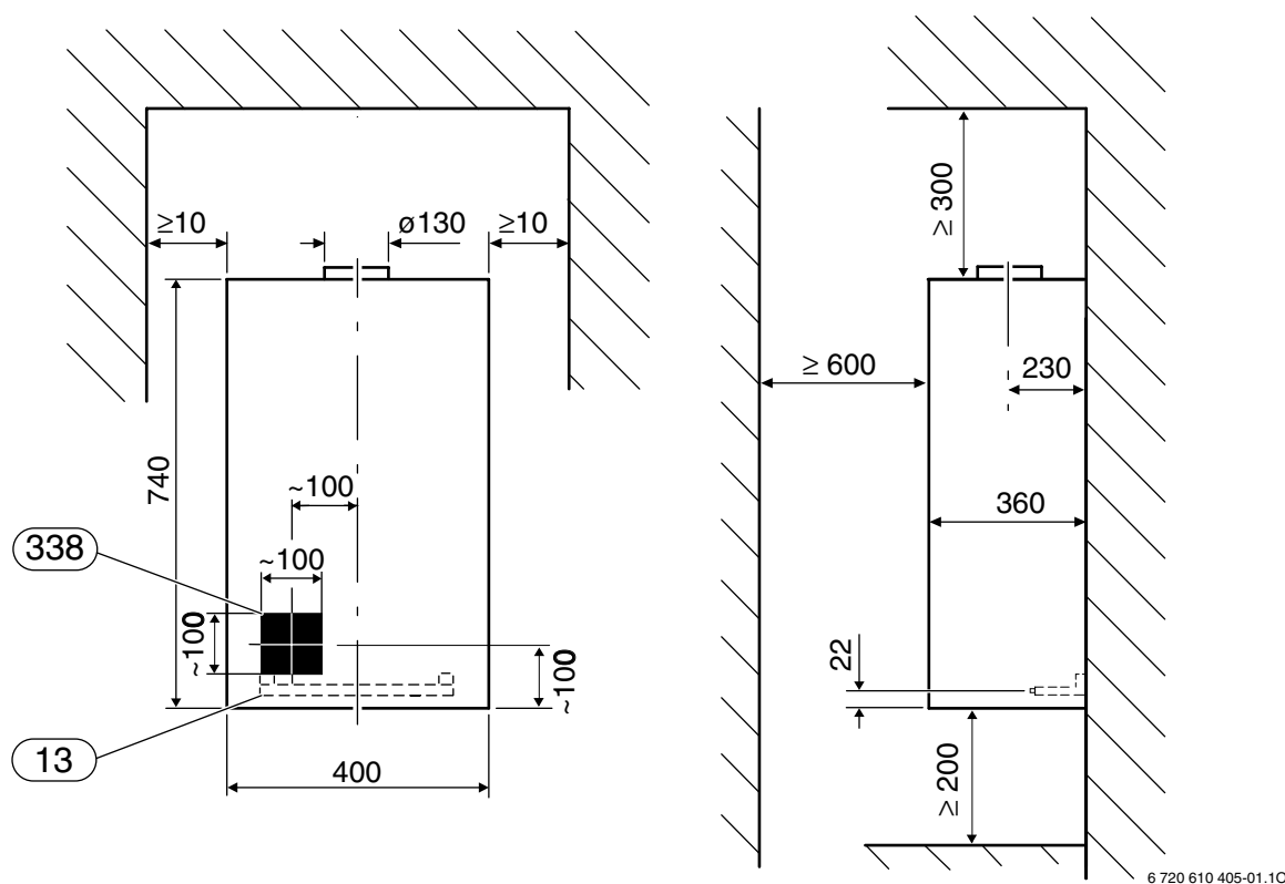
obr. 1 Pohled zepředu a z boku
