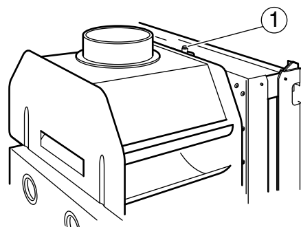
obr. 19 Automatické odvzdušňování
