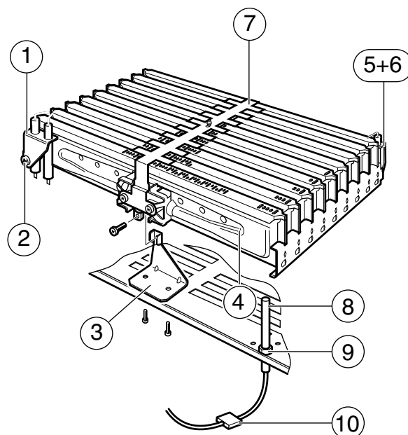
obr. 40 Sestava hořáku
