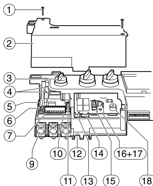
obr. 11 Připojení na modulu
