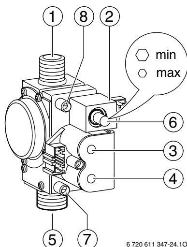
obr. 24 Plynový ventil
