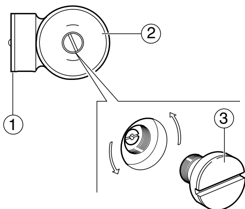
obr. 20 Odvzdušnění/odblokování čerpadla
