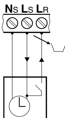
obr. 16 Připojení programovací jednotky (odstraňte propojku mezi LS a LR)
