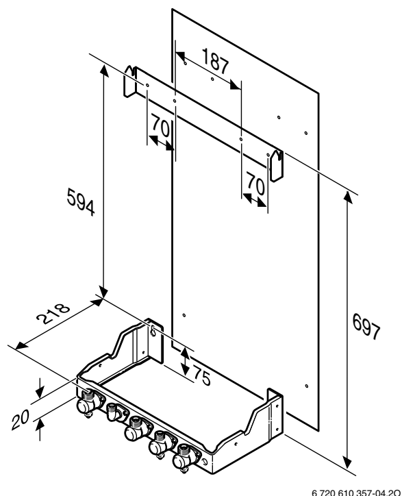
obr. 5 Sestava pro montáž na zeď
