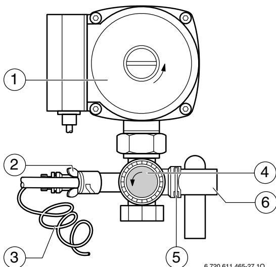
obr. 21 Připojení odtoku pojišťovacího ventilu
