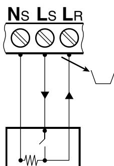
obr. 15 Připojení pokojového termostatu 230 V (odstraňte propojku mezi LS a LR)
