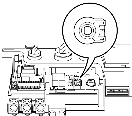
obr. 26 Nastavení maximálního tepelného výkonu pro ústřední vytápění
