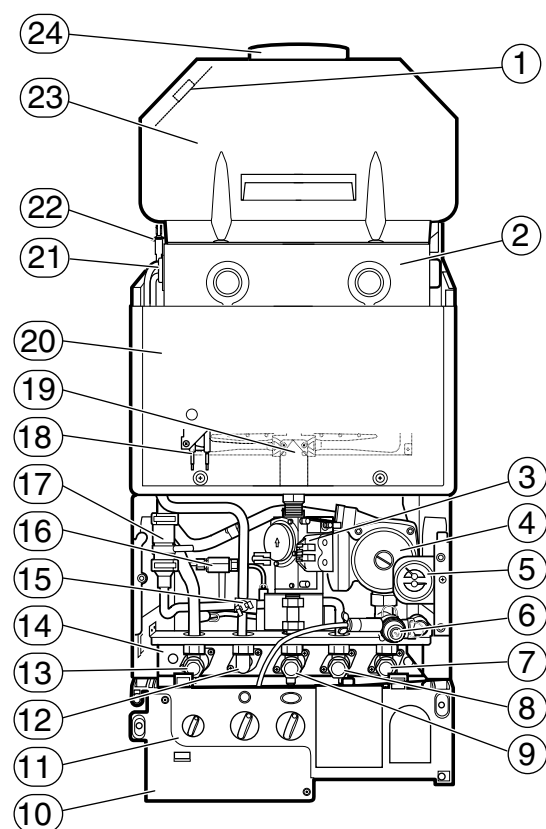
obr. 18 Schéma kotle s modulem v servisní poloze
