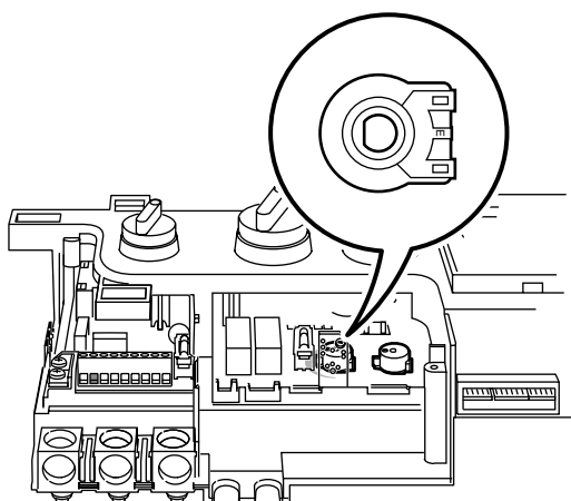
obr. 22 Nastavení režimu ovládání čerpadla
